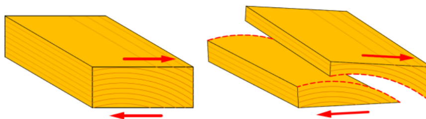
Figura 1.3 - Mecanismo de ruptura de lamela por rolling shear
