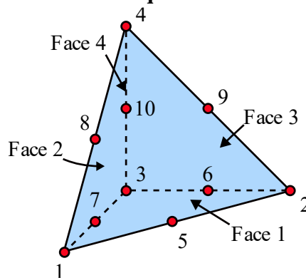
Figura 3.8 - Elemento tetraédrico quadrático com 10 nós do tipo C3D10
