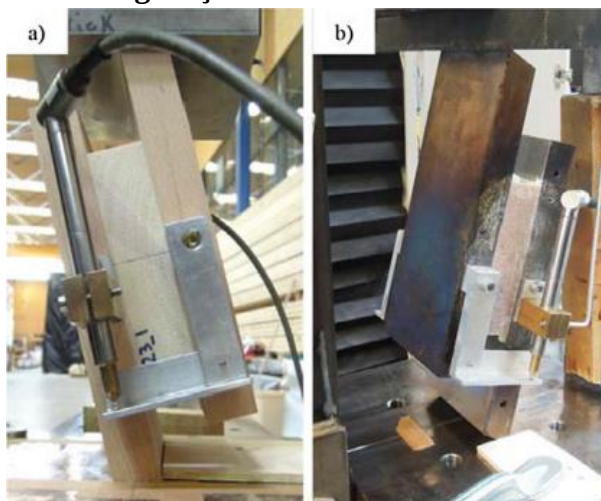
Figura 2.28 - Configuração do teste de cisalhamento modificado
