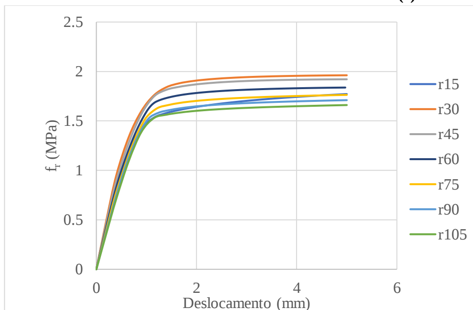
Figura 4.9 - Diagrama de tensão de rolling shear ( f_r ) e deslocamento para diferentes valores de distância da medula ao centro da lamela ( r )
