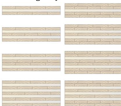
Figura 2.16 - Configurações das camadas de MLCC
