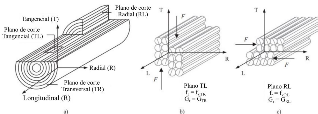
Figura 2.23 - Eixos principais do tronco (a) e planos de rolling shear TL (b) e RL (c)
