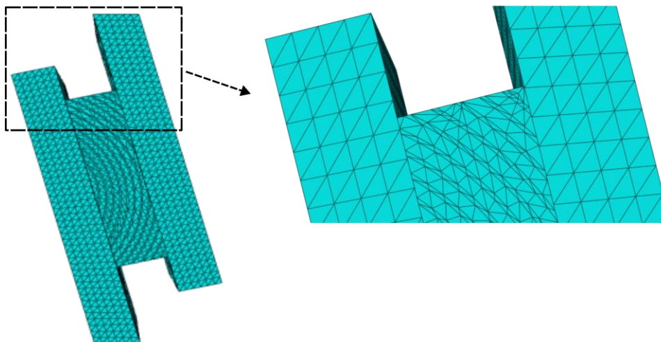
Figura 3.9 - Configuração da malha
