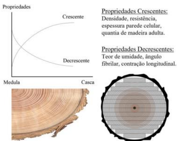
Figura 2.5 - Propriedades da madeira juvenil dentro do tronco e com cortes de tábua
