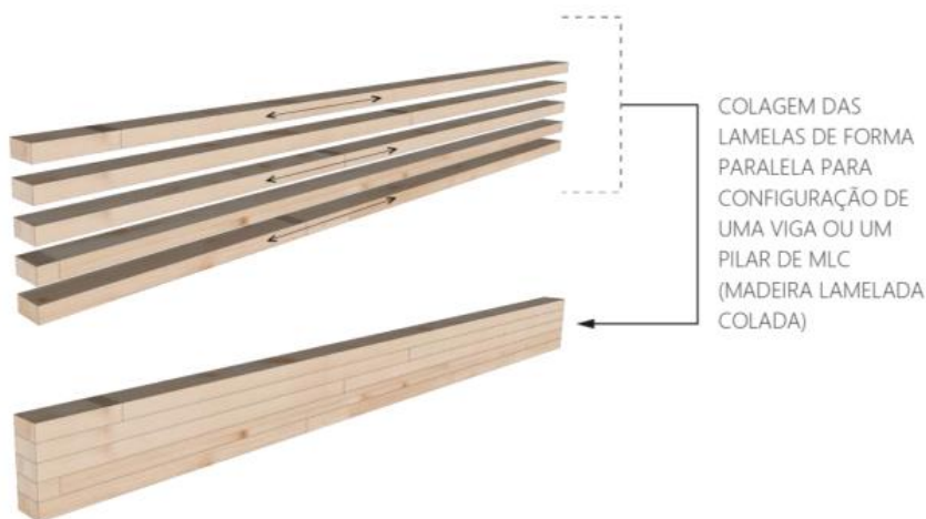
Figura 2.15 - Madeira Lamelada Colada
