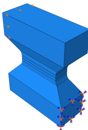
Figura 3.4 - Condições de contorno do ensaio de cisalhamento utilizado na validação
